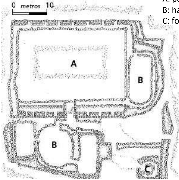
Ruinas de los Quilmes Planta de casa comunal.
